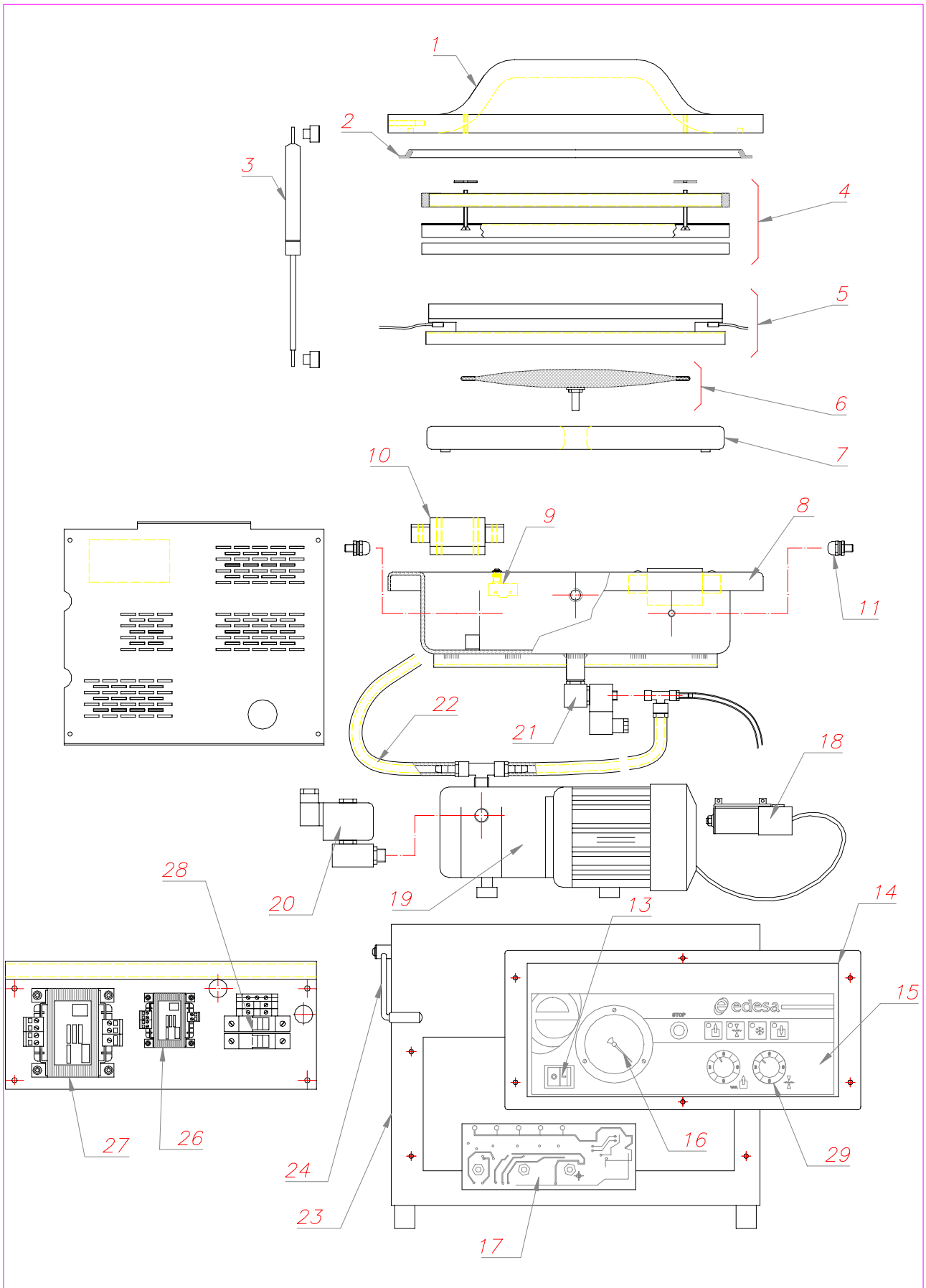
Envasadora al vacío VAC-6 T
